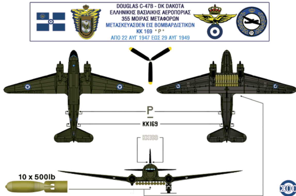
Γραμμικό διάγραμμα τριών (03) όψεων του υπό Διακριτικών Νηολογίου Κλήσεως (ΔΝΚ): ΚΚ-169 (P) μετατραπέντος Βομβαρδιστικού Douglas C-47/DC-3 «Dakota», όπως αυτό δημιουργήθηκε από τη μελέτη και ανάλυση σχεδίων, φωτογραφιών και εγγράφων κειμένων από τον ιστορικό Νικόλαο Δημητριάδη (Αρχείον ΕΕΕΣ Α.Ε. «Κηρύκειον»).
